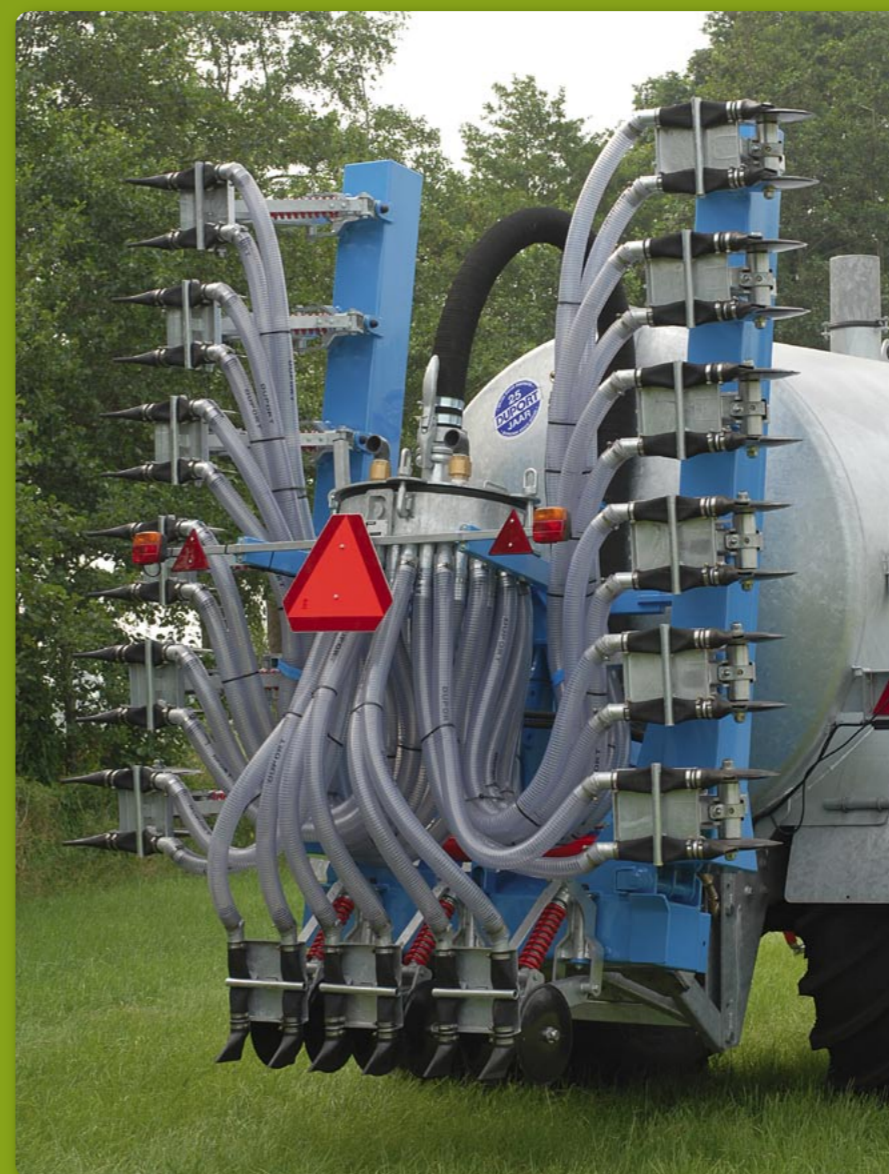
Afsluitmechanisme-farmer
